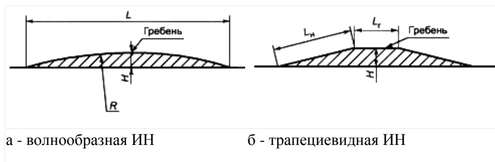
Рисунок 1 - Поперечные профили ИН
